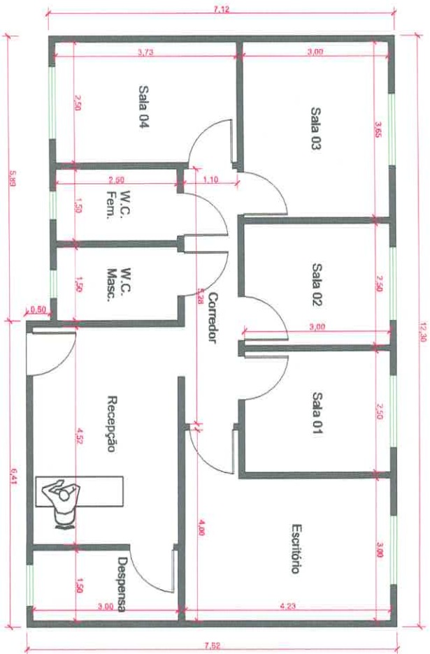
PLANTA BAIXA ÁREA TOTAL: 90,78m²
