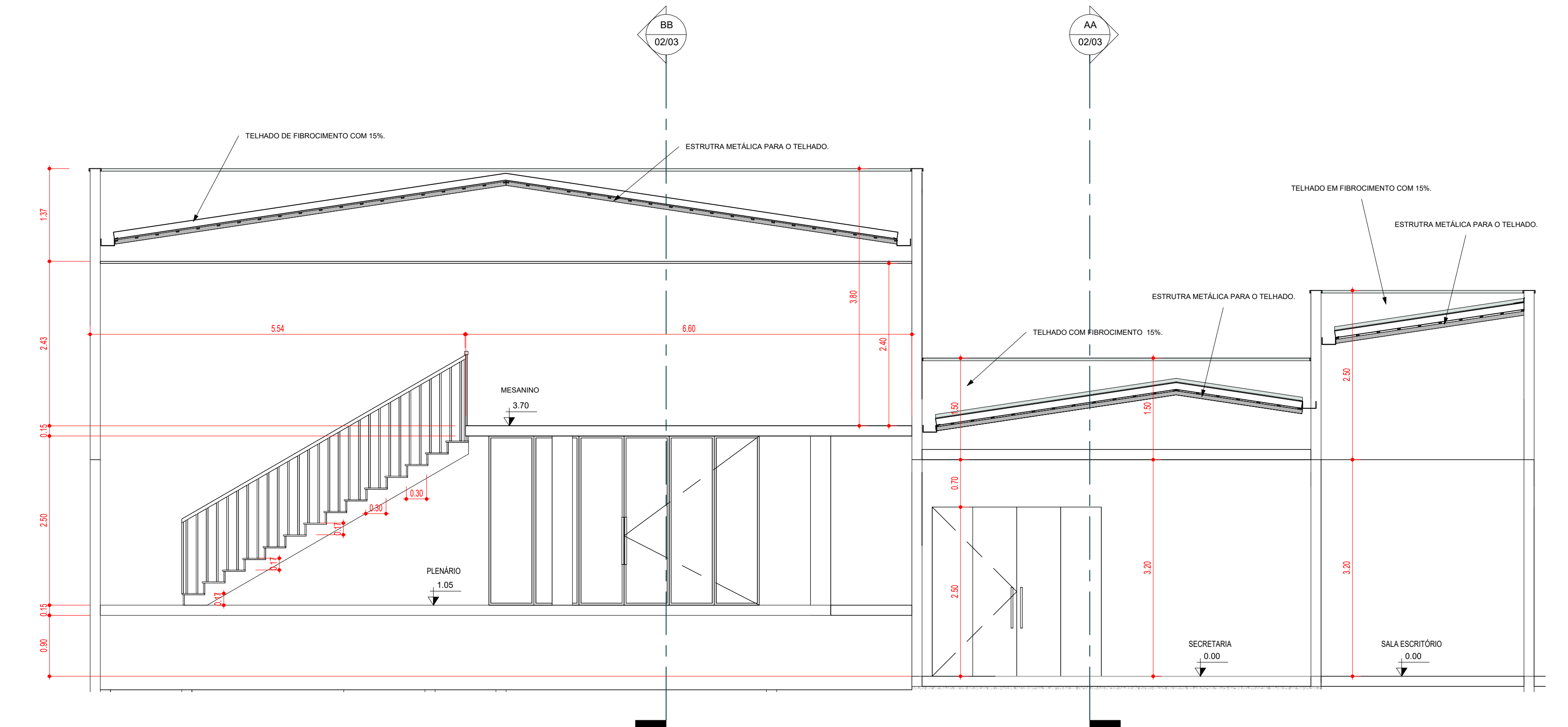
DD CORTE DD 1:50
