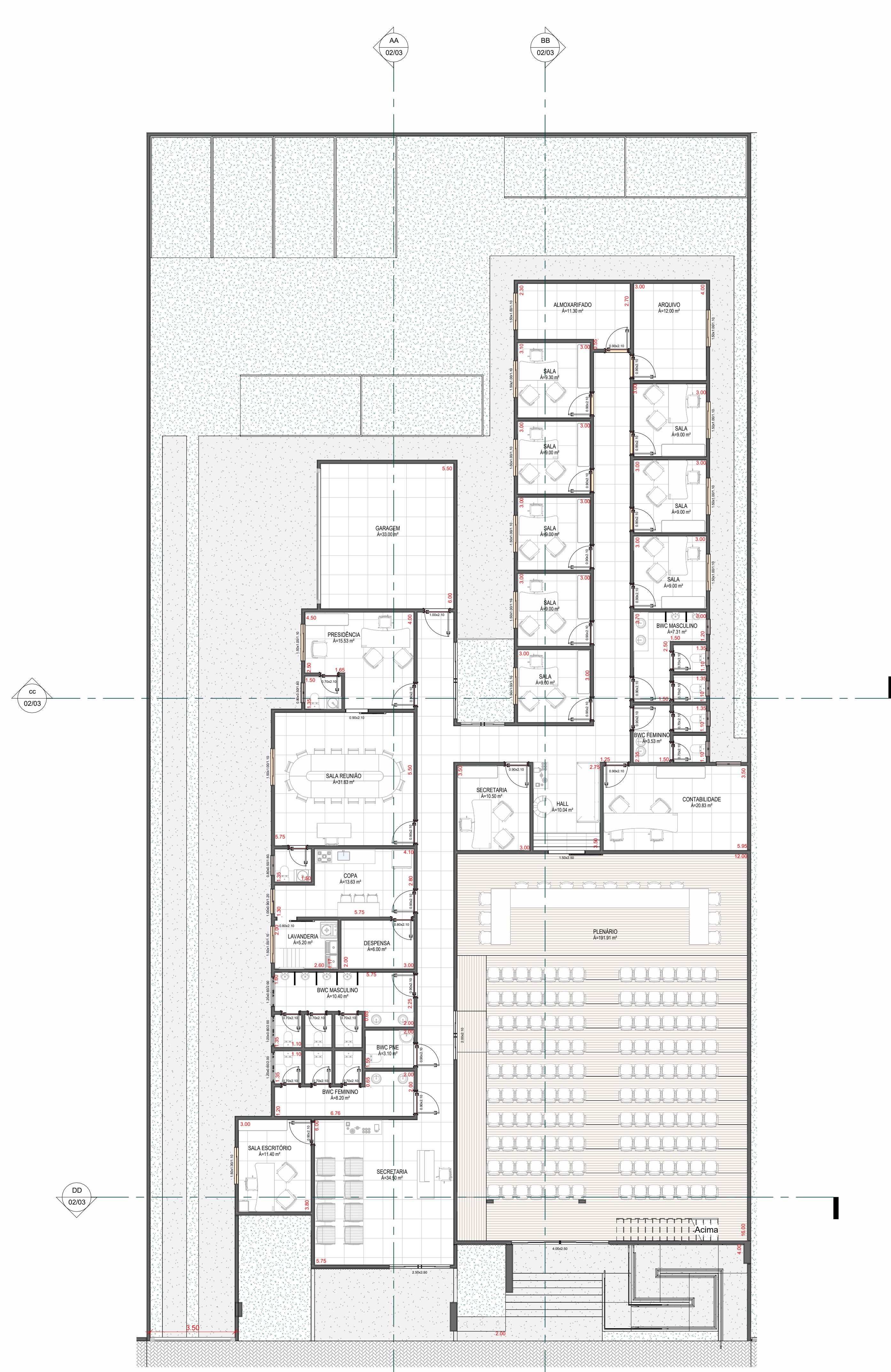
2 PLANTA LAYOUT 1:100
