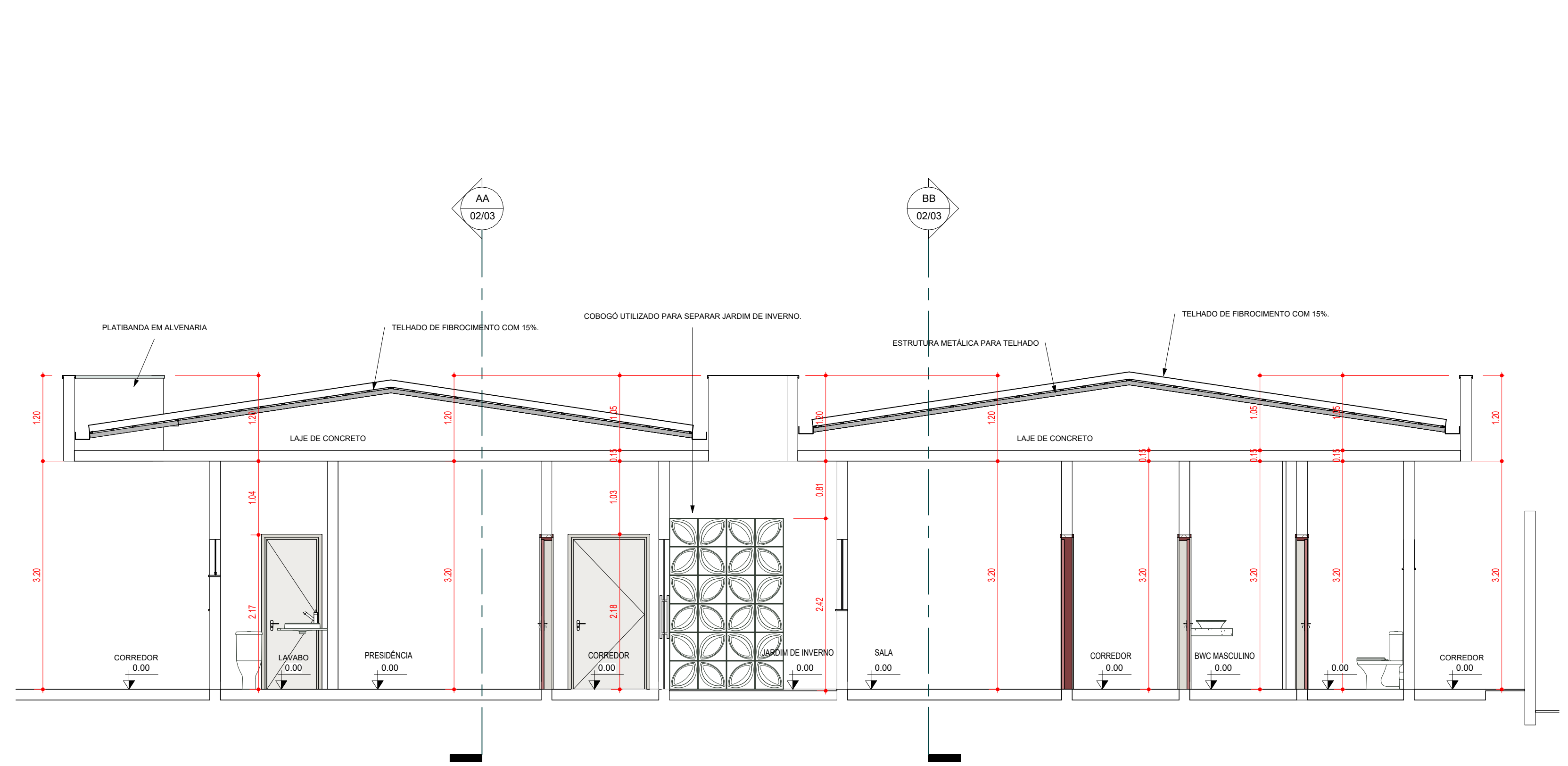
CC CORTE CC 1:50
