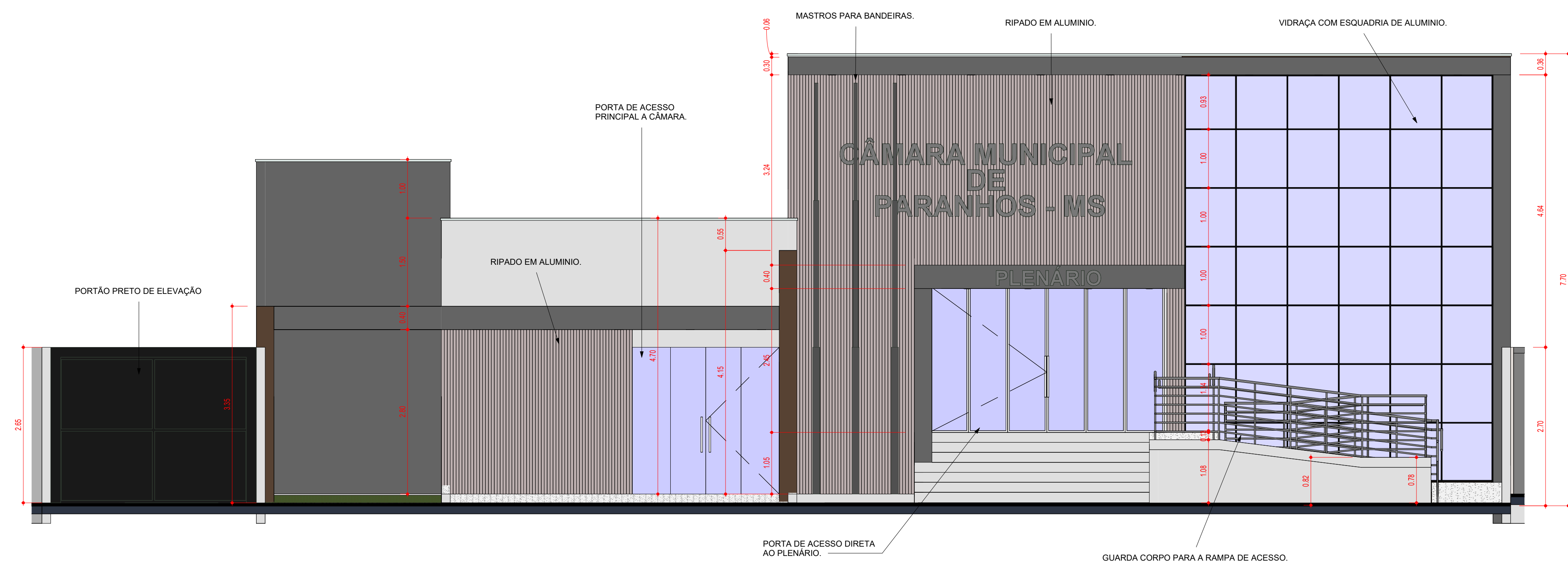
1 VISTA FRONTAL 1:50
