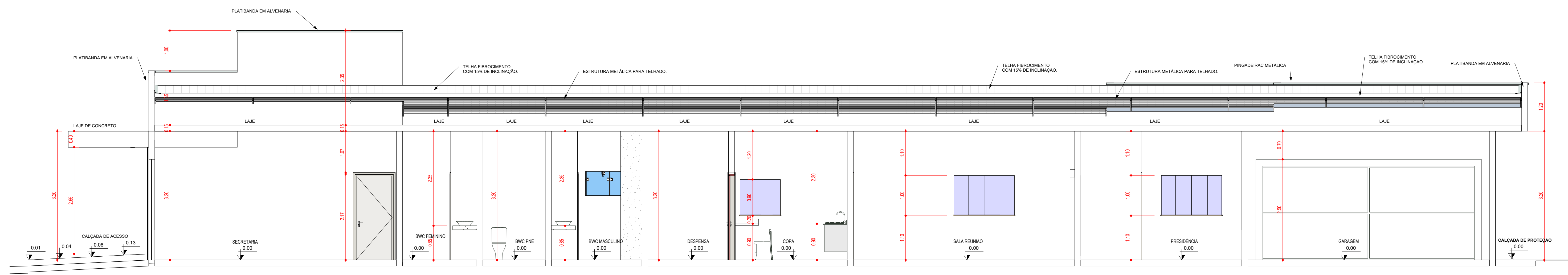
AA CORTE AA 1:50
